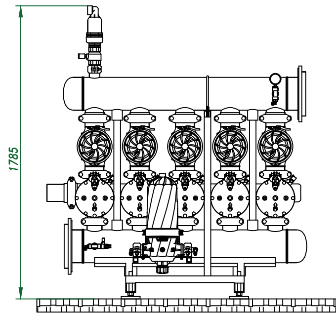
Вид спереди
